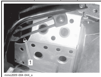
1. Резиновый фиксатор
