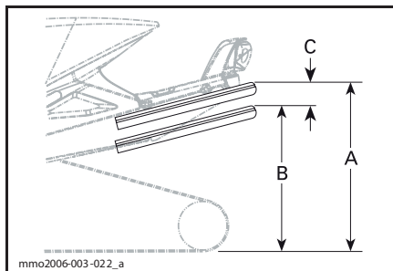
A. Максимально растянутая подвеска B. Подвеска под нагрузкой (вес водителя, пассажира и груза) C. Разница между величинами «А» и «В» не должна превышать 50 мм - 75 мм; обратитесь к таблице
