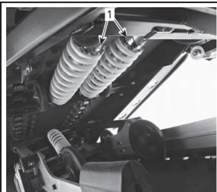
СДВОЕННЫЙ АМОРТИЗАТОР 1. Регулировка задних пружин
