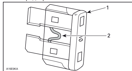
1. Предохранитель 2. Плавкая вставка, которую нужно проверить
