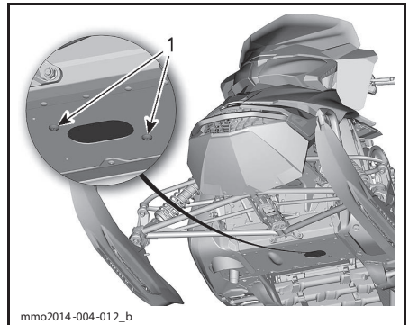
ПОВЕРНИТЕ СЕРВИСНУЮ КРЫШКУ 1. Фиксирующие винты
