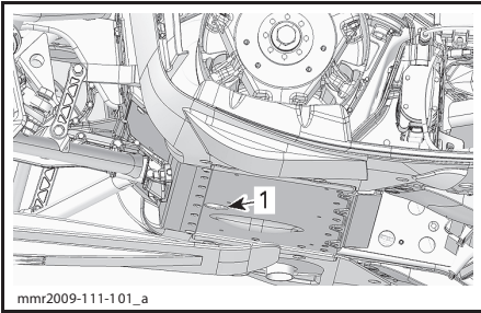
1. Отверстие в раме для доступа к сливной пробке
