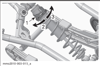
ТИПОВОЙ ВАРИАНТ ТИП РЕГУЛЯТОРА - АМОРТИЗАТОР С ГАЗОВЫМ ПОДПОРОМ ВЫСОКОГО ДАВЛЕНИЯ (HPG™)
