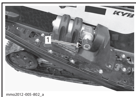
ВИД СПРАВА 1. Регулятор силы демпфирования медленно-го/быстрого сжатия
