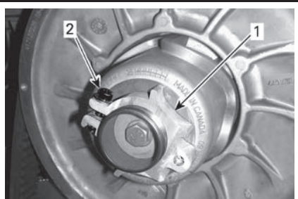
1. Регулировочная муфта 2. Фиксирующий болт
