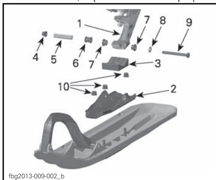
fbg2013-009-002_b СХЕМА РАСПОЛОЖЕНИЯ ДЕТАЛЕЙ – ПОКАЗАНА ПРАВАЯ СТОРОНА
