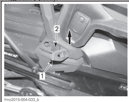
1. Резиновый выступ 2. Фиксатор LINQ
