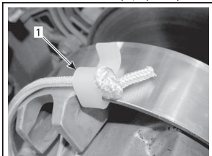
1. Место установки зажима
