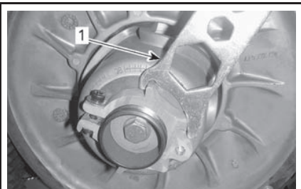
1. Ключ для регулировки подвески
