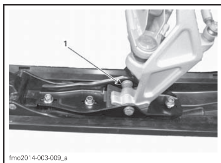
fmo2014-003-009_a 1. Втулка с внутренней стороны лыжной стойки
