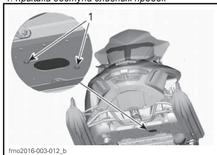
ПОВЕРНИТЕ КРЫШКУ ДОСТУПА 1. Винты крепления
